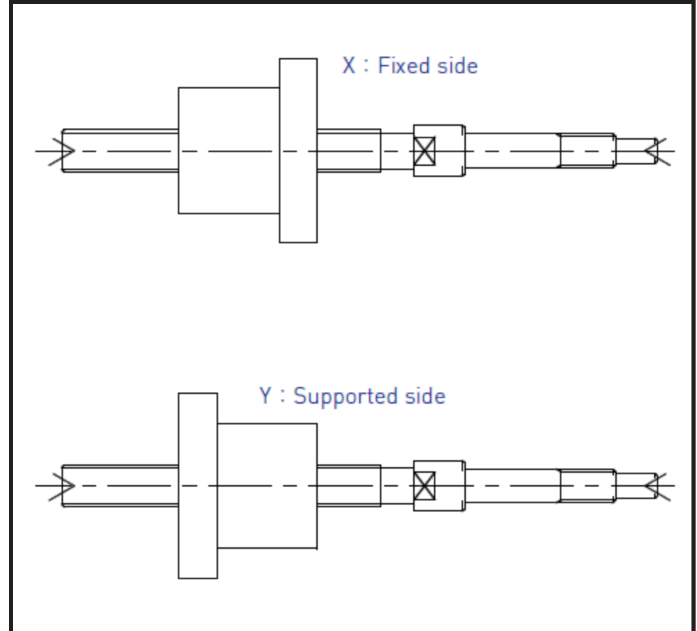
Fig. A-23 : Nut Flange direction
