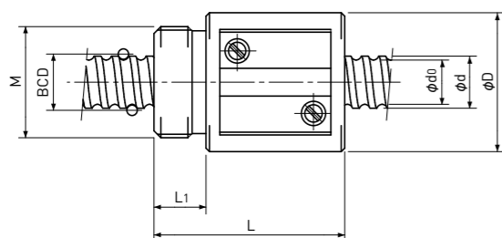
Type-1:Return-plate type
