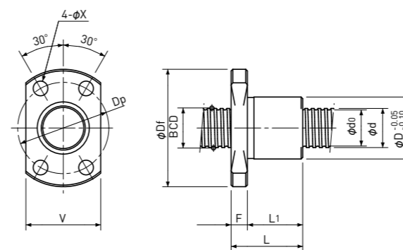
Type-2:End-deflector type
