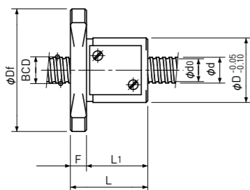
Type-1:Return-plate type
