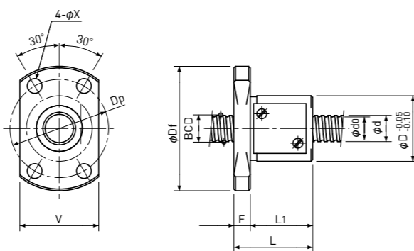
Type-1:Return-plate type
