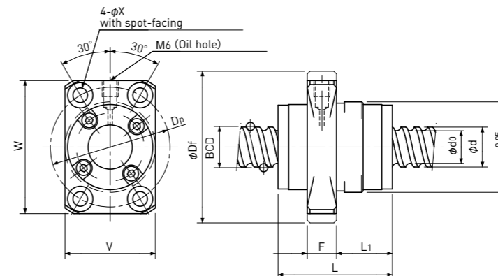
Type-4:End-deflector type
