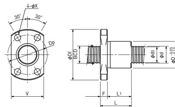
Type-2:End-deflector type
